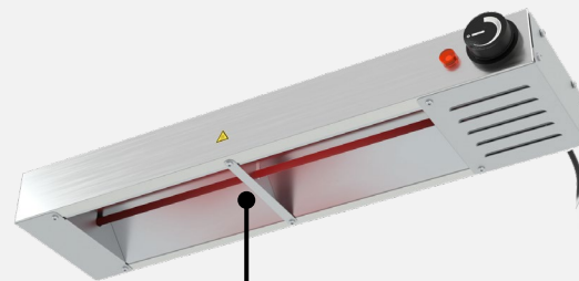
Calrod element with high IR emissivity for better thermal efficiency Resistenza lineare ad alta emissività di IR per una miglior efficienza termica
